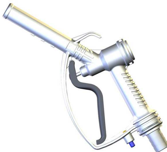
PMP120 B Pistola Plastica Bianca Travaso gasolio/prodotti chimici Guarnizioni in VITON Interni in PP+FV+INOX
